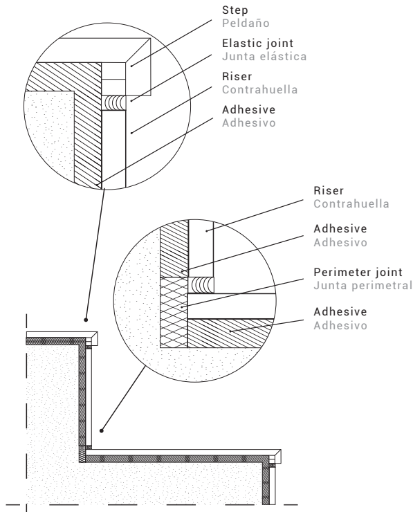
Detail of peldaños en escalera (UNE 138002:2017) Detalle de peldaños en escalera
